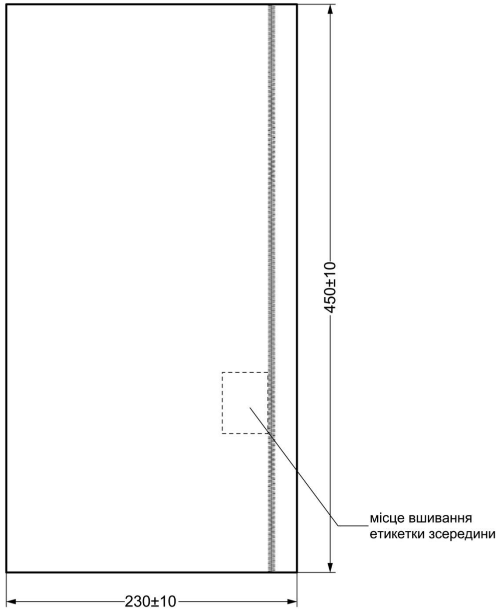
Рисунок Б1.1– Лінійні виміри виробу
